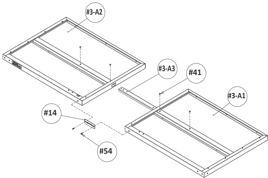
(#3-A) Top Panel
