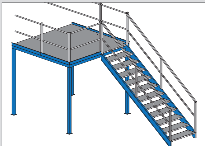
Einläufige gerade Treppen
