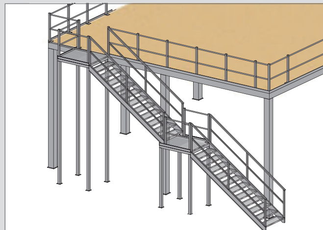
Zweiläufige gerade Treppen mit Zwischenpodest
