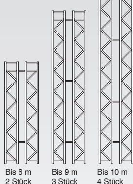
Anzahl Distanzstücke in der Höhe
